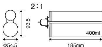
カートリッジ装着図
